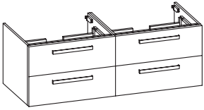
Waschtischunterschrank mit Siphonausschnitt 4 Auszüge
