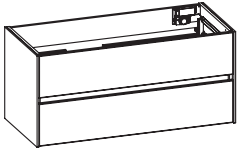
Waschtischunterschrank inkl. LED-Profil mit Bewegungssensor für Griffjungen 2 Auszüge, Kosmetikeinsatz im oberen Auszug, 2-teilig
